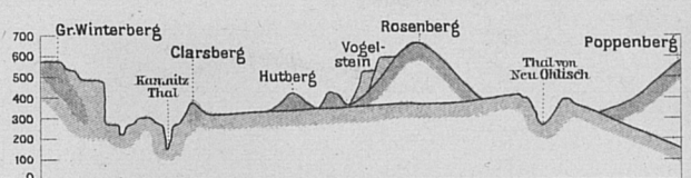
Profil vom Winterberg über den Rosenberg zum Poppenberg.
