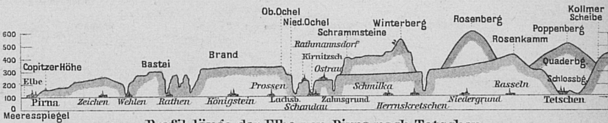
Profil längs der Elbe von Pirna nach Tetschen. Maßstab der Länge 1 : 400.000, M. d. Höhe 1 : 40.000.
