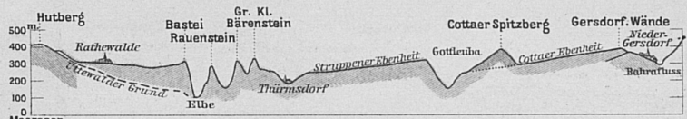
Profil von Rathewalde über die Bastei und den Cottaer Spitzberg nach Nieder-Gersdorf.
