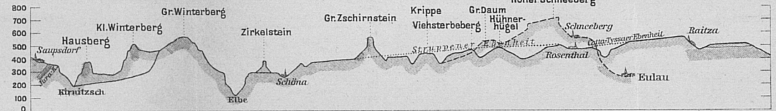
Profil von Saupsdorf über die Winterberge, den Gr. Zschirnstein u. den Schneeberg nach Raitza.
